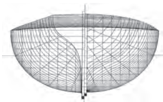
Spantenriss
